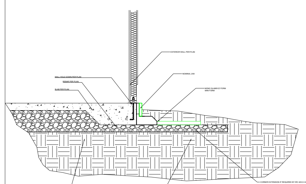
2- UNHEATED SPACE
