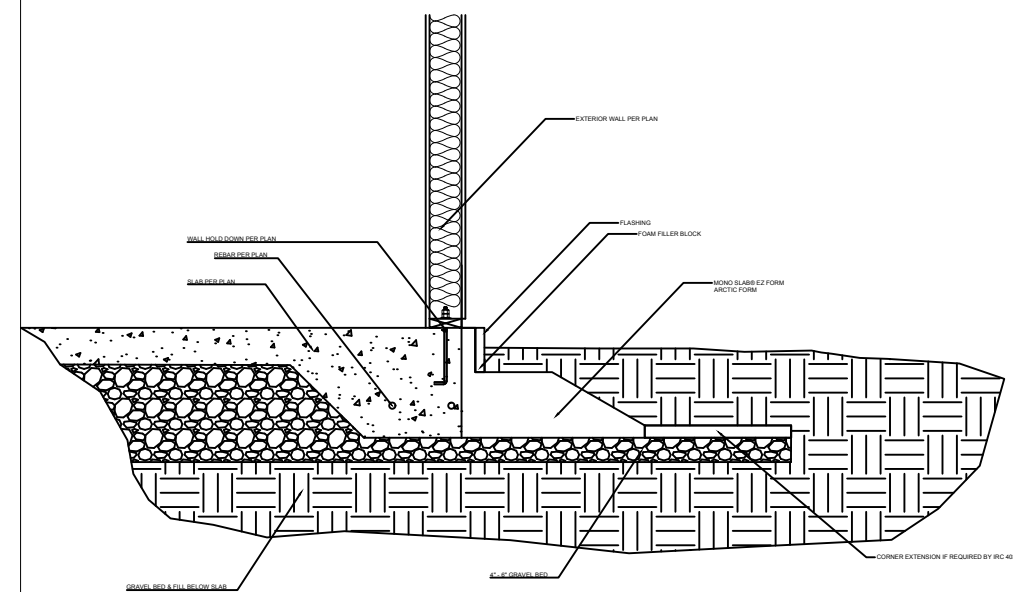
2- UNHEATED SPACE
